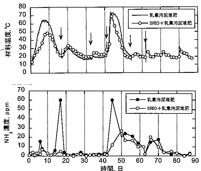
図 1 堆肥温度と NH 3 揮散量の変化 (矢印は切り返し)
